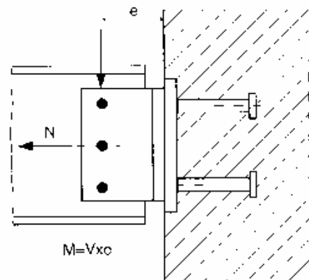
Anschluß Stahlträger an einbetonierter Ankerplatte
